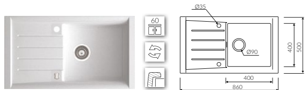
PROFIR 860 1KO Index: 160 113 0xx L 860 W 500 H 230 mm
