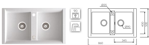
PROFIR 860 2K Index: 160 203 0xx L 860 W 500 H 230 mm
