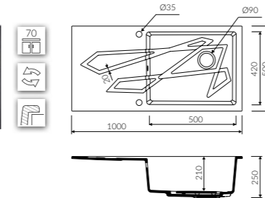
FOORN II 1000 1KO Index: P_Z_034_11_1000 L 1000 W 500 H 250 mm
