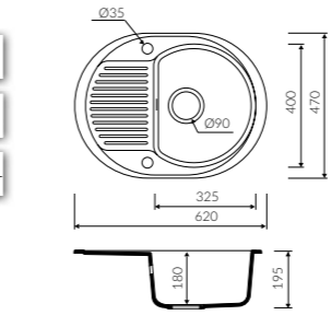
DURO 620 1KO Index: P_Z_025_11_0620 L 620 W 470 H 195 mm
