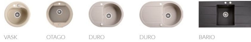
VASK OTAGO DURO DURO BARIO
